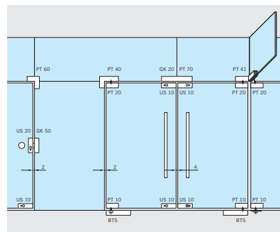
14 Technische Details
